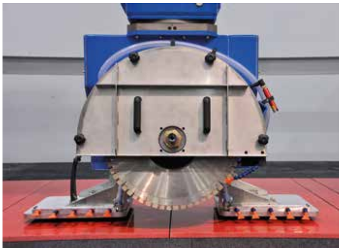
Manipulador de ventosas con capacidad de hasta 500 kg (opcional 1000 kg para modelos Brembana Sprint y Brembana Gixa), para garantizar la manipulación de piezas de piedra de gran grosor.
